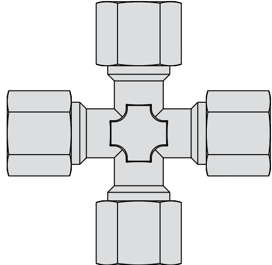
43-0000-09 接头, 十字型, 8 mm
