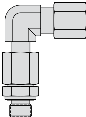
43-0000-13 弯头, 旋转, 6 mm-G1/8 双头螺柱
