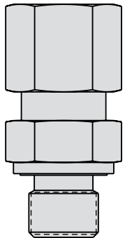
43-0000-12 连接, 标准, 8 mm-G1/4 双头螺柱
