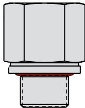
30-8782-64 外丝 G1/4 - 内丝 SAE 4
