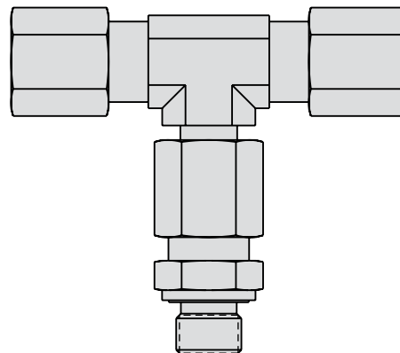
43-0000-15 T型, 分流, 旋转, 6 mm-G1/8 双头螺柱
