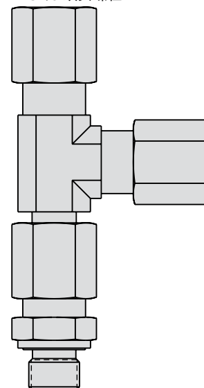
43-0000-17 T型, 三通, 旋转, 6 mm G1/8 双头螺柱
