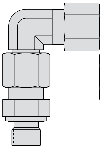
43-0000-14 弯头, 旋转, 8 mm-G1/4 双头螺柱
