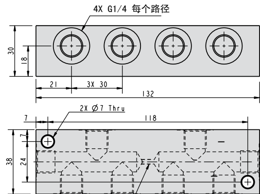
要改变成8孔单路径, 最小钻孔Ø5mm, 直通
