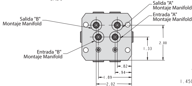
Válvula Check Piloteada "A-B" Circuito Modelo No. 70-3311-12 ILS703301 REV A
