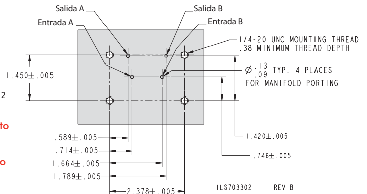
Dimensiones de Montaje para Válvula Check A-B Modelo No. 70-3311-12
