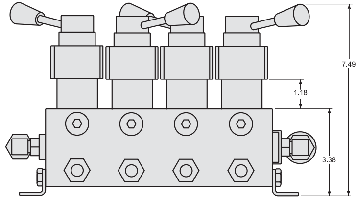
Planos de Control 4 Válvulas
