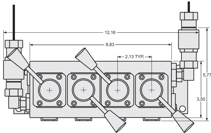
Planos de Control 4 Válvulas
